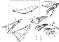
Plástica Trasera
