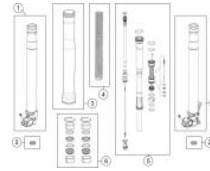
Horquilla delantera
