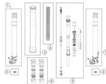
Repuestos horquilla delantera
