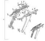
Chasis trasero
