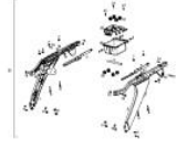
Chasis trasero
