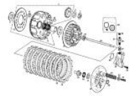
EMBRAGUE
