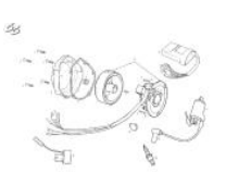
Generador 125
