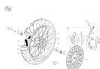
Rueda delantera SM
