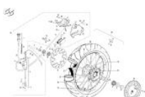
Rueda trasera SM
