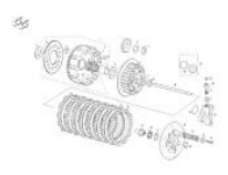
Embrague 200-250-300
