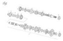
Cambio 200-250-300
