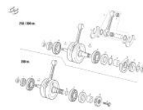
Cigüeñal 200-250-300
