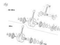
Cigüeñal 200-250-300
