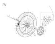
Rueda delantera EC-MX
