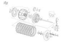
Embrague 200-250-300
