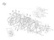
Carter de motor 200-250-300
