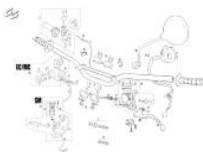
Manillar - mandos
