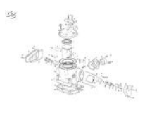
Cilindro 200-250-300
