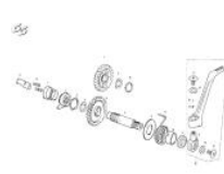
Palanca de arranque 200-250-300
