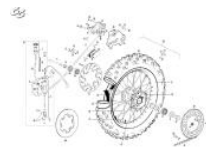
Rueda trasera EC-MX
