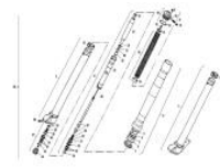
Horquilla delantera marzocchi EC 250-300
