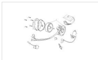
Generador 125
