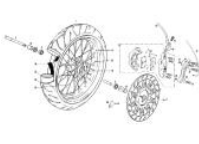
Rueda delantera SM
