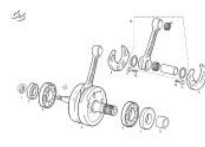
Cigüeñal 125
