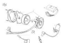
Generador 200-250-300
