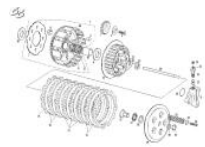
Embrague 125
