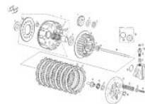
Embrague 200-250-300
