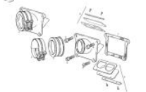
Válvula de láminas 125
