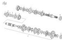
Cambio 200-250-300
