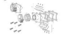
Válvula de láminas 200-250-300
