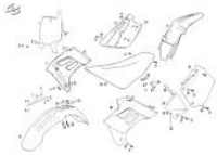
Carrocería MX
