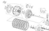
Embrague 200-250-300
