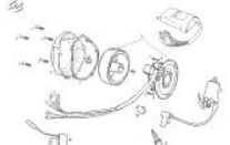
Generador 125
