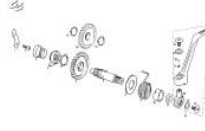
Palanca de arranque 125
