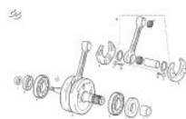
Cigüeñal 125
