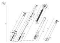
Horquilla delantera Marzocchi
