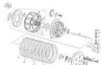
Embrague 125
