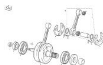
Cigüeñal 125
