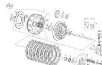
Embrague 200-250-300
