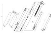
Horquilla delantera marzocchi EC-SM
