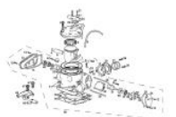
Cilindro 200-250-300
