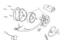
Generador 125
