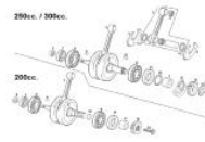
Cigüeñal 200-250-300
