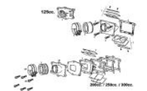
Válvula de láminas
