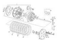
Embrague 125
