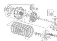
Embrague 200-250-300
