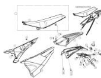
Plástica Trasera
